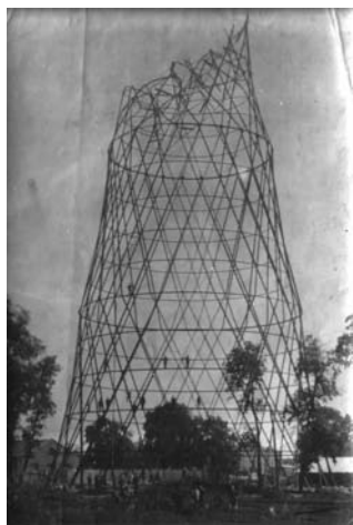
Июль 1921г. Шабаловская башня после аварии
